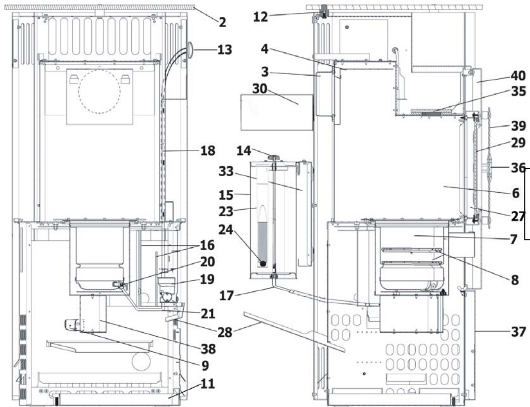
Abbildung 2: Ölofen Ibiza 469.50
