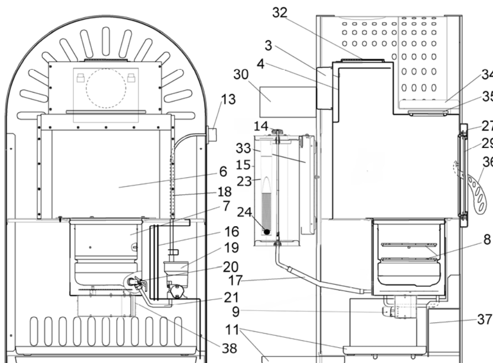
Abbildung 1: Öfen Viking 468.50
