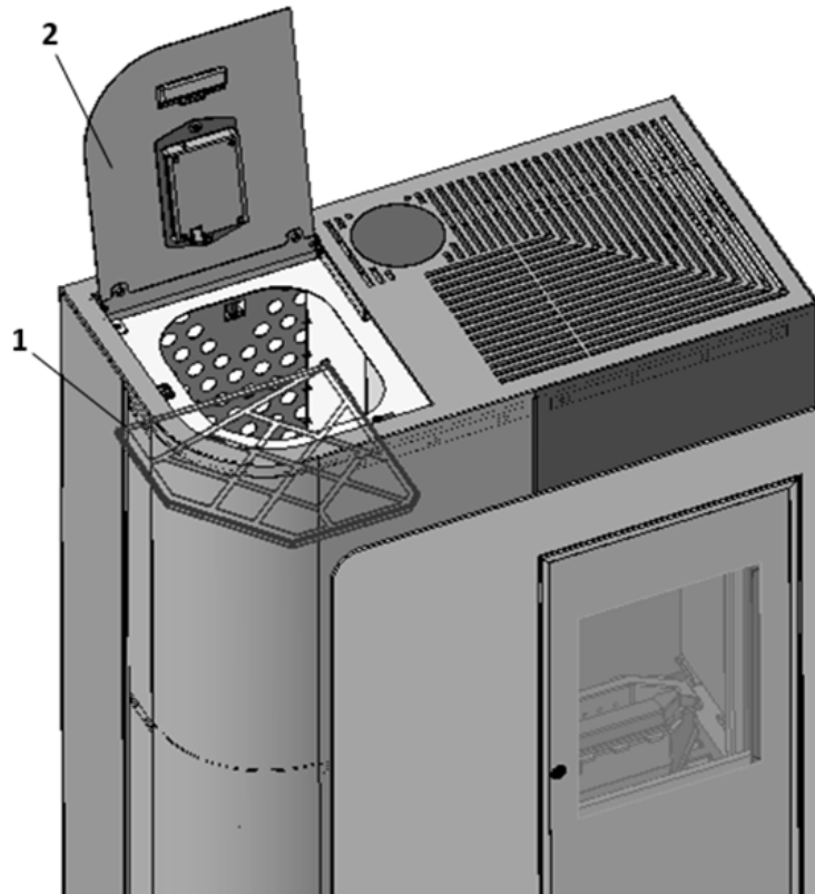
Abbildung7: Pellettank
