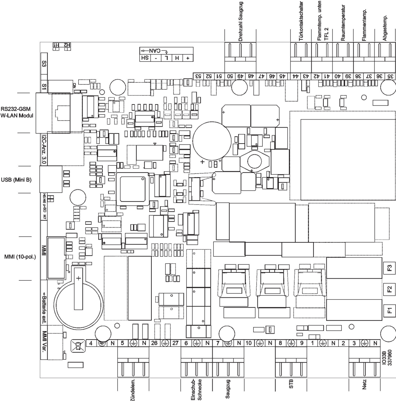
Anschlussplan IO 33.3
