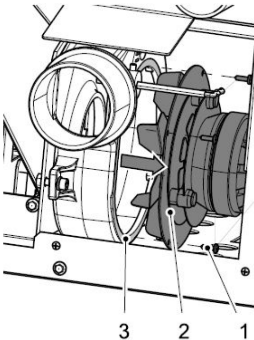
Abbildung 9: Saugzuggebläse
